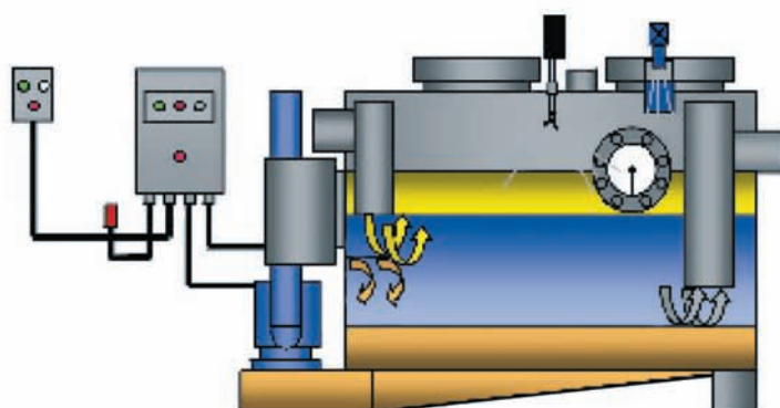
Комплектация 4 с прямым отводом для очистки, насосом для шлама, внутренней очисткой высоким давлением и автоматическим управлением
