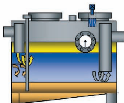
Комплектация 2 с прямым отводом для очистки
