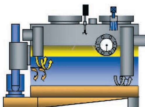
Комплектация 3 с прямым отводом для очистки, насосом для шлама, внутренней очисткой высоким давлением и ручным управлением
